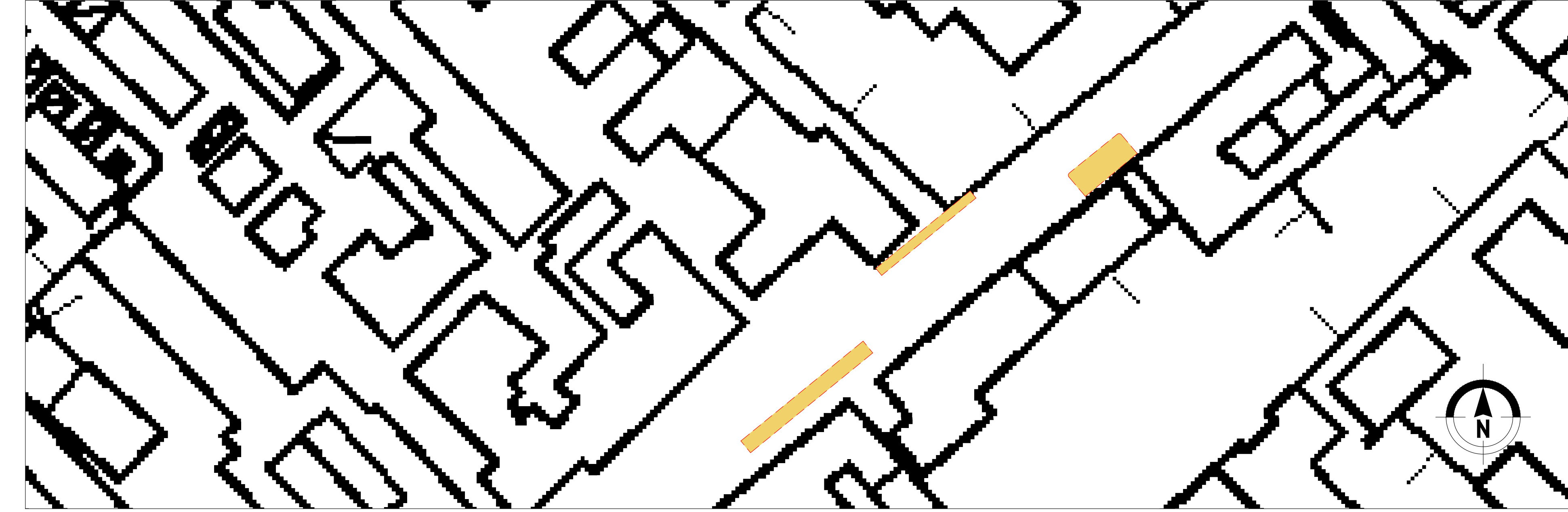
1 BARICELLA - SCALA 1:500
